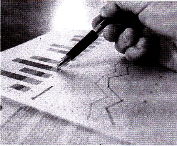
Gambar 2.2 Menyiapkan data
